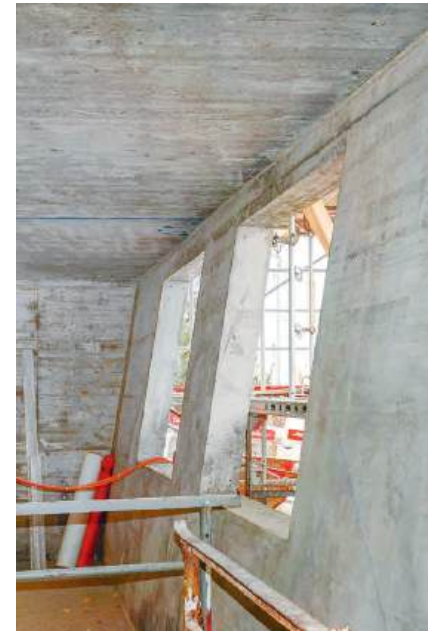
Die gleiche Fassade vom inneren Wohnraum, Abweichung 60cm aus der Vertikalen
