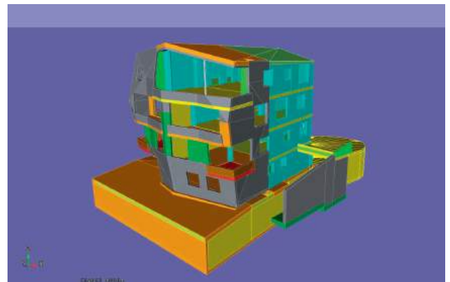
Visualisierung des Objektes. Jede Etappe weist eine andere Abweichung aus der Vertikalen auf. Im Erdgeschoss ca. 60cm und im Dachgeschoss zum Teil über einen Meter.
