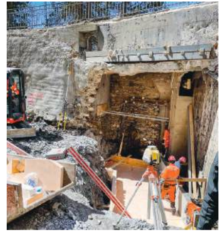
Der spätere Eingang führt durch die Bruchstein Aussenmauer. Wir sicherten das Mauerwerk mittels Stahlträgern
